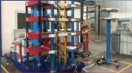
600kV impact body
